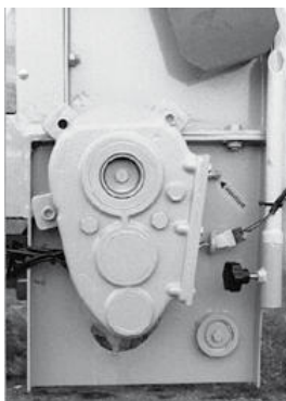
Гидропривод цепи
